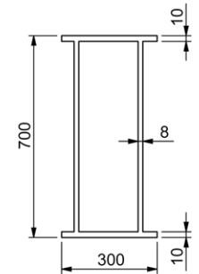
Mặt cắt dầm chính
